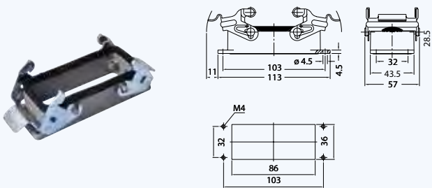
32x16A - 12x35A Makine Gövde
