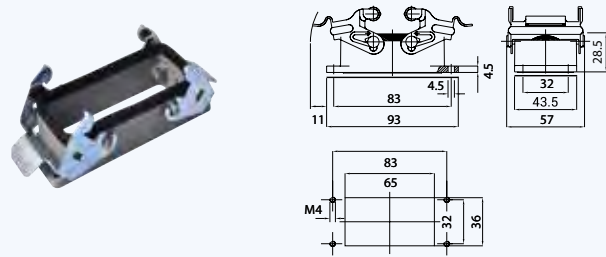
24x16A Makine Gövde
