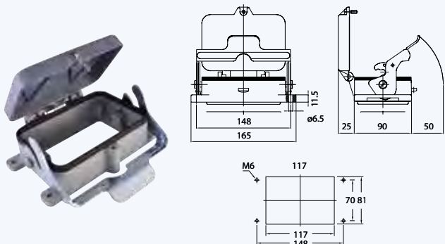
48x16A Makine Gövde
