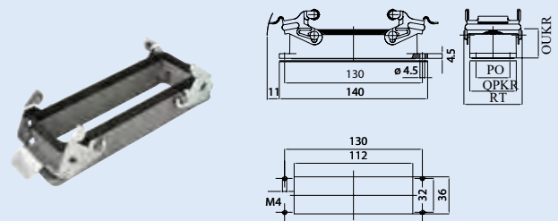
48x16A Makine Gövde
